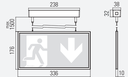
R32S SEILMONTAGE
