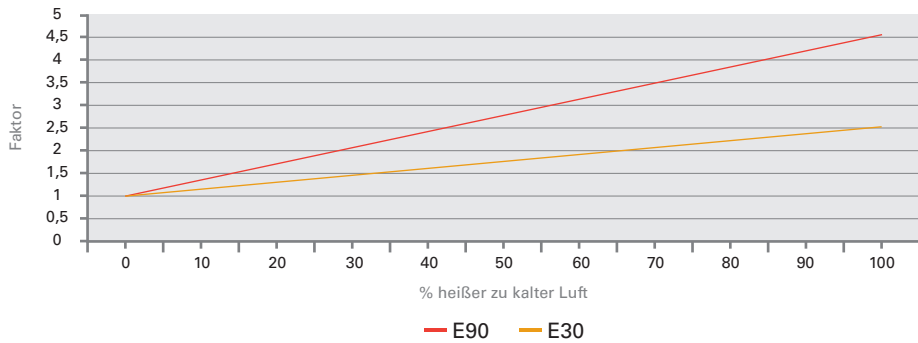
Querschnittsermittlung E30/E90
