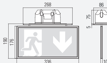
R32E DECKENEINBAUMONTAGE
