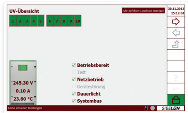
Übersicht der angeschlossenen Unterstationen
