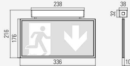
R32E DECKENEINBAUMONTAGE
