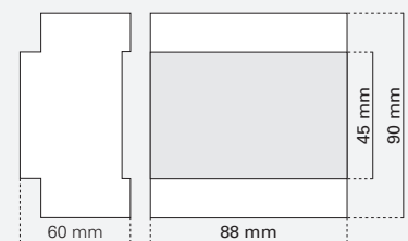
Hutschienenmontage 5 TE
