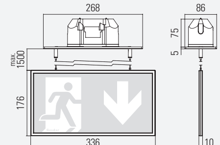
R32F SEILEINBAUMONTAGE
