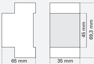
Hutschienenmontage 2 TE
