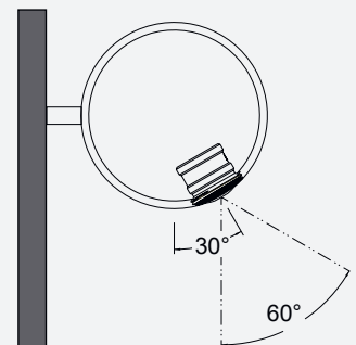
SYMMETRISCHE LINSE 501* Einseitig abstrahlend
