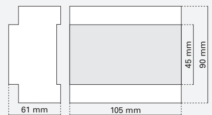
Hutschienenmontage 6 TE
